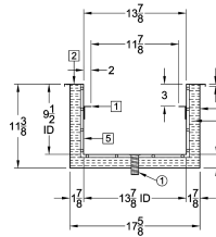
SECTION THRU SCALE: 1"=1'
